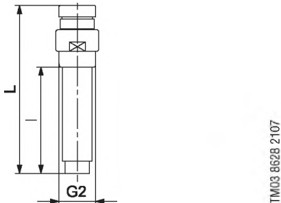
Рис. 25 Стандартный вариант исполнения, DN 32
