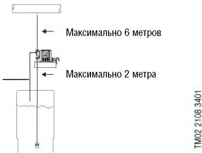
Рис. 2 Максимальная длина трубок
