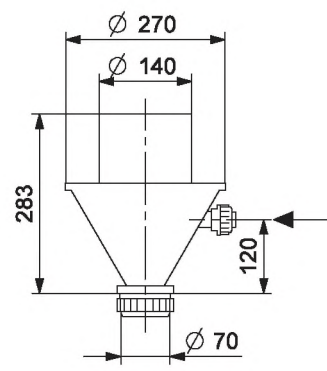
Рис. 58 Загрузочная воронка для приготовления растворов
