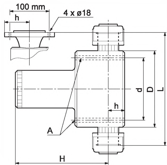
Рис. 45 Размеры, DN 32
