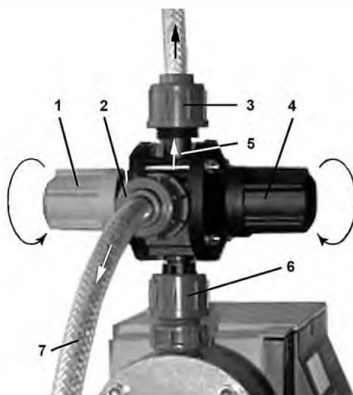
Рис. 47 Многофункциональный клапан
