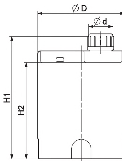
Рис. 54 Резервуар, 1 000 литров
