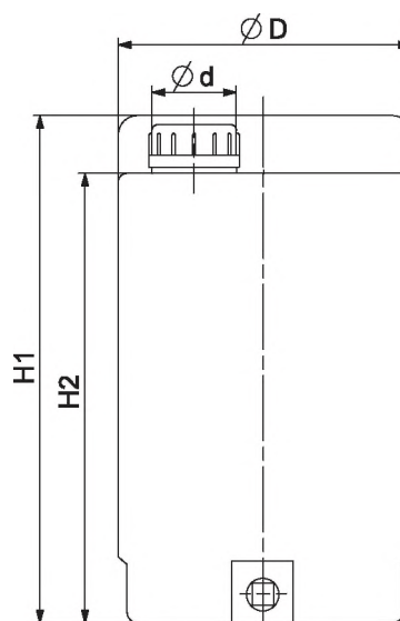
Рис. 52 Резервуар, 75 литров
