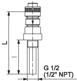
Рис. 23 Стандартный вариант исполнения, с использованием нержавеющей стали и сплава Hastelloy
