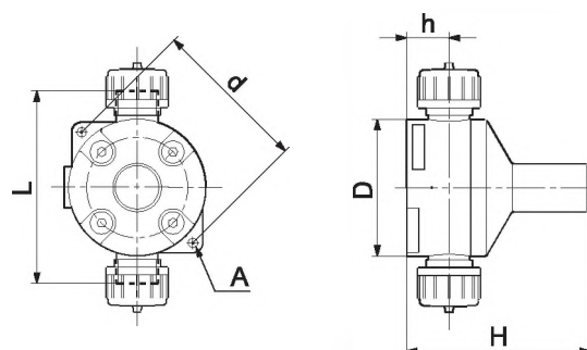
Рис. 41 Размеры, DN 4/DN 8
