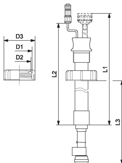
Рис. 15 Жесткая всасывающая линия для канистр
