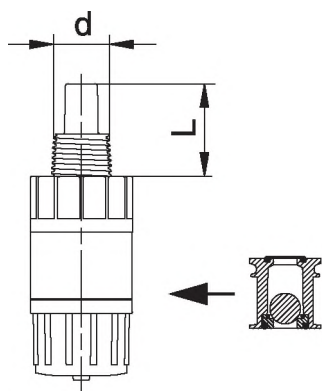
Рис. 17 Размеры инжекционного клапана, производительность до 60 л/ч
