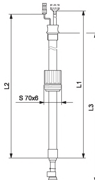
Рис. 14 Жесткая всасывающая линия для сменных резервуаров
