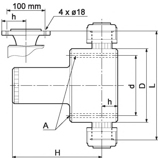
Рис. 43 Размеры, DN 20
