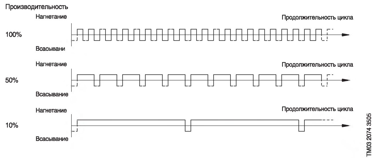
Рис. 4 Соотношение между скоростью нагнетания и производительностью
