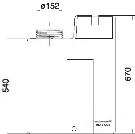
Размеры [мм]
