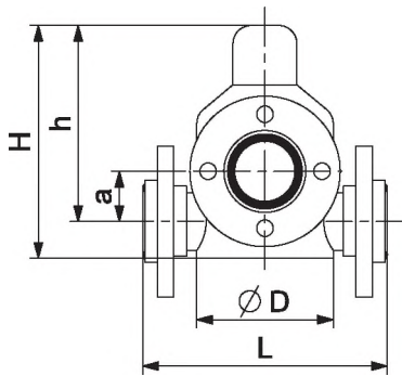
Рис. 39 Клапан сброса давления, DN 65
