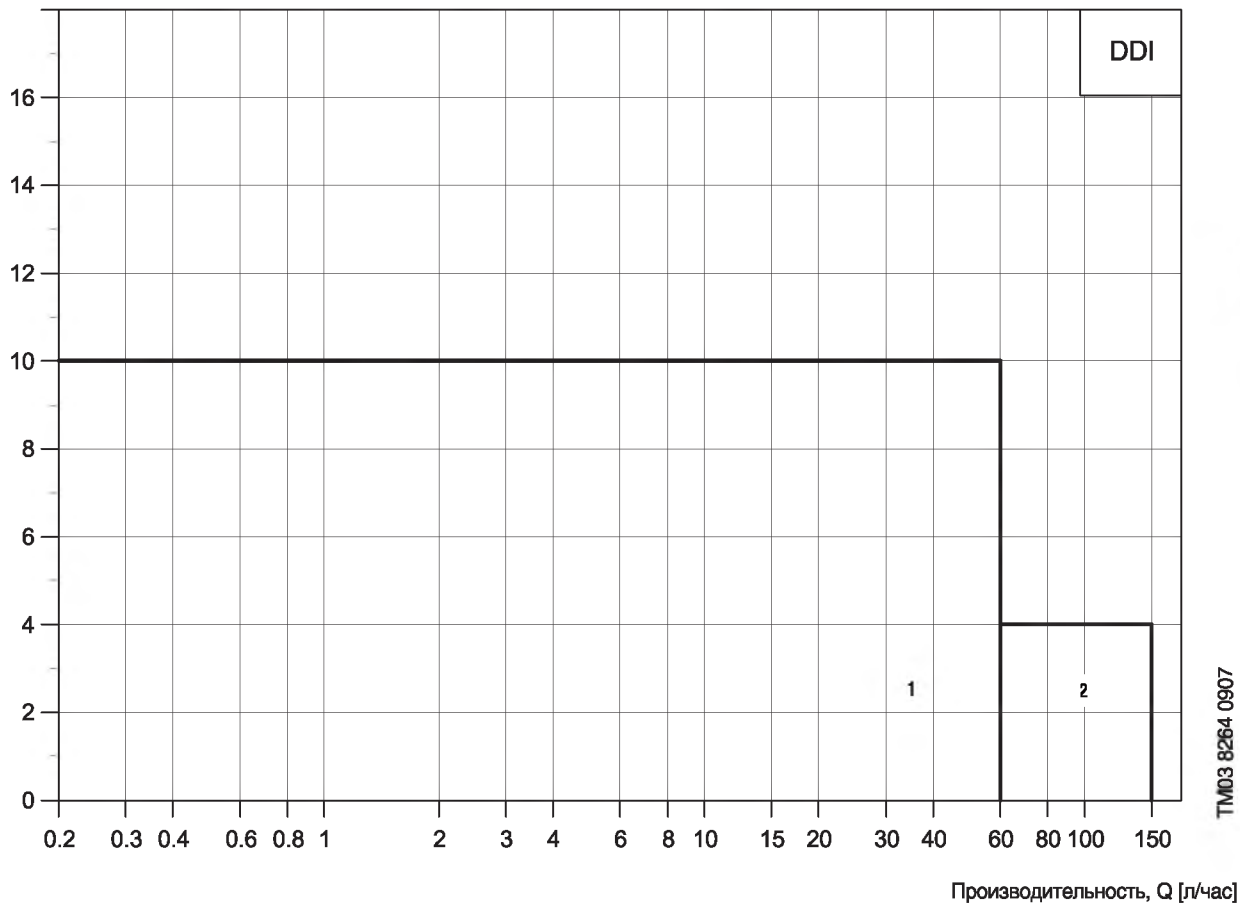
Рис. 2 Диапазон производительности, насос DDI
